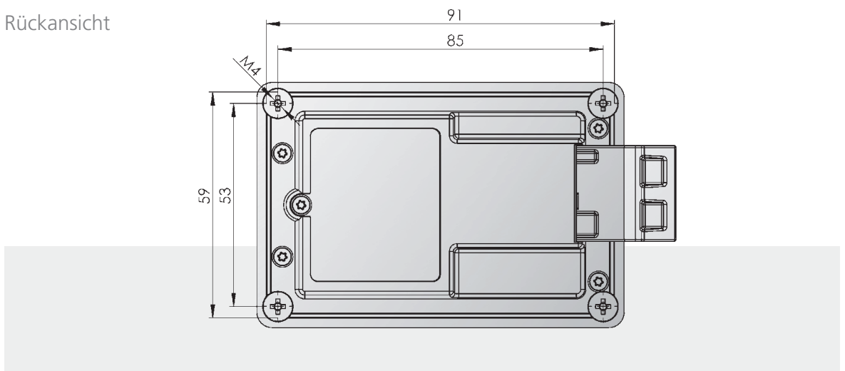
Draufsicht
